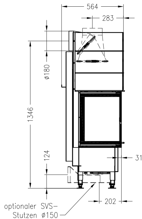
Seitenansicht M~1:20
