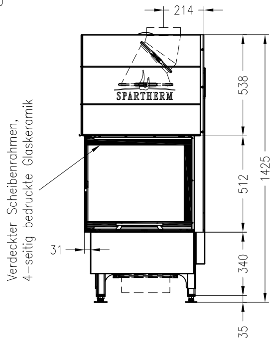
Vorderansicht M~1:20
